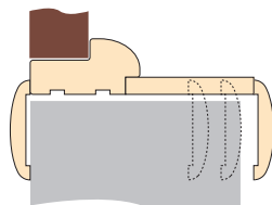
Схема устройства дверных проёмов
