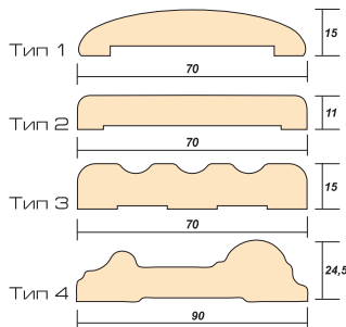
Наличник Сращенный массив сосны, шпон дуба
