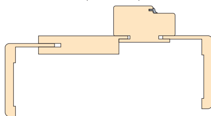
Коробка в сборе
